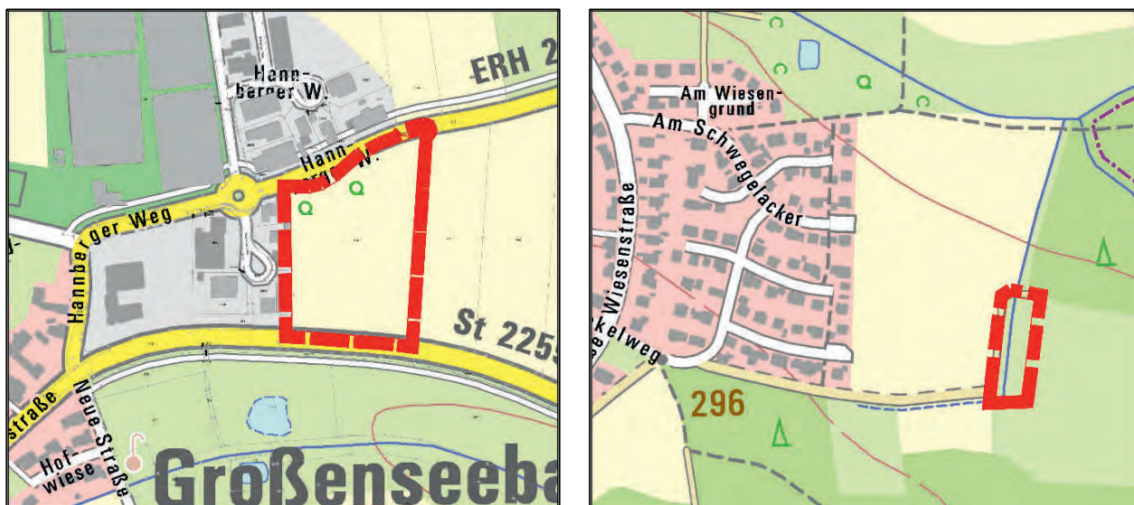
Lageplan des räumlichen Geltungsbereiches des Bebauungsplans (links) sowie der zugeordneten Ausgleichsfläche o. M. (Kartengrundlage Geobasisdaten © Bayerische Vermessungsverwaltung 2024)
